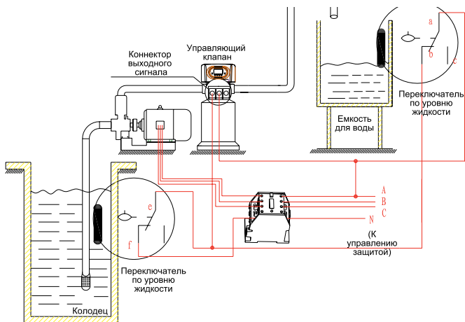
Рис. 3-6 Схема электрических соединений Переклюателя по уровню жидкости в емкости для воды, контролирующего работу насоса на входе в систему.
